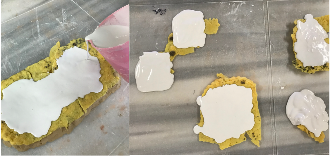
Görsel 4. Silikon modeller üzerine refrakter kalıp karışımının dökülmesi (Kaynak: Yazarın kişisel arşivi)
