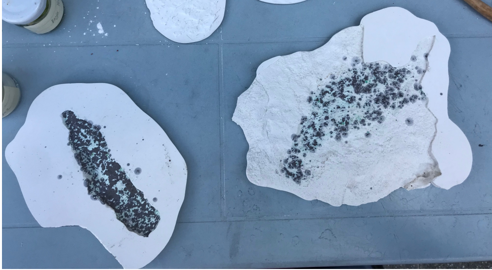
Görsel 6. Refrakter kakıp üzerine yardımcı malzemelerin uygulanması (Kaynak: Yazarın kişisel arşivi)
